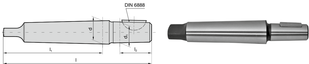
Kegeldorn DIN 238 mit Scheibenfeder DIN 6888 Arbor DIN 238 with woodruff key DIN 6888
